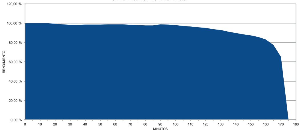
GRÁFICA DESCARGA - RGBWA-UV A 100%
