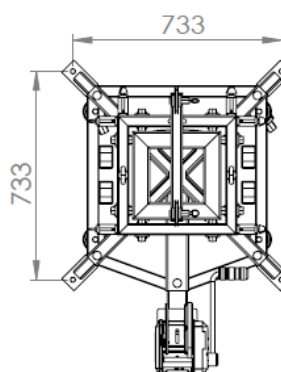
Anclajes al suelo / Floor anchorage
