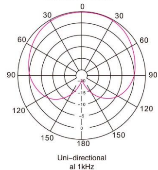
Patrón Polar
