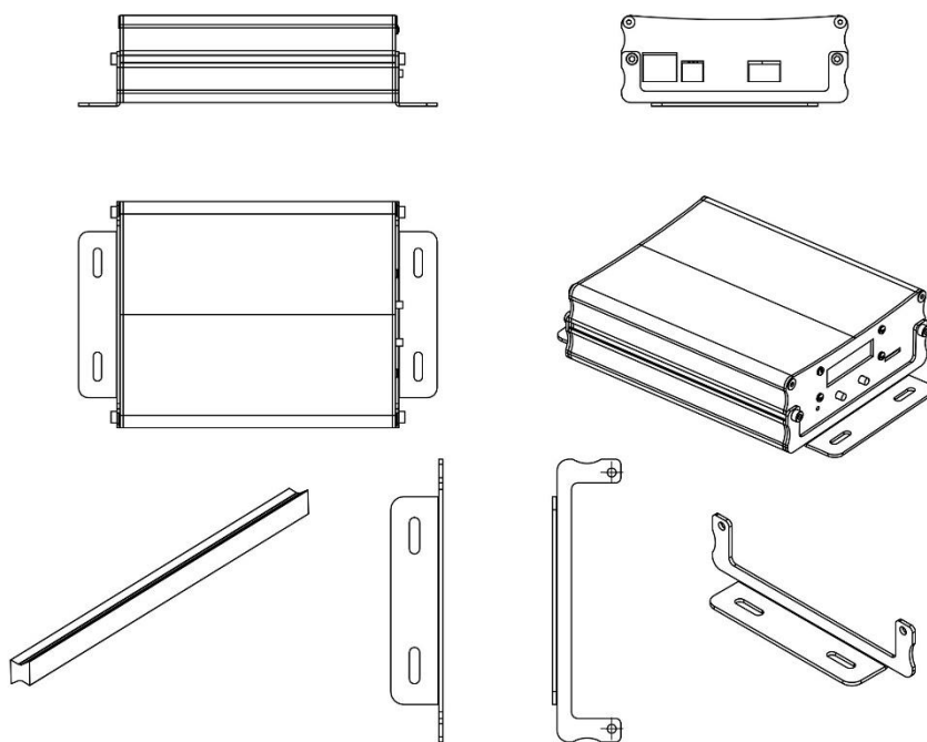
1x Fixation bar to joint two WPE devices (WPE24/WPE44) 1x Barra de fijación para unir dos dispositivos WPE (WPE 24/WPE44)
