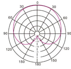
Patrón Polar
