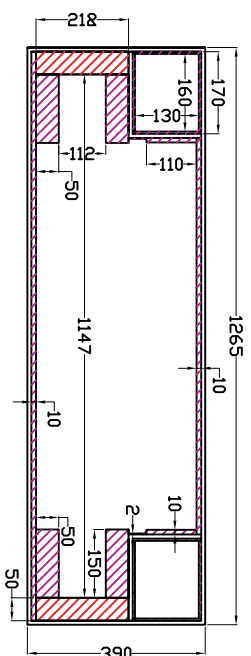
SECTION D-D
