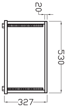
D-D
